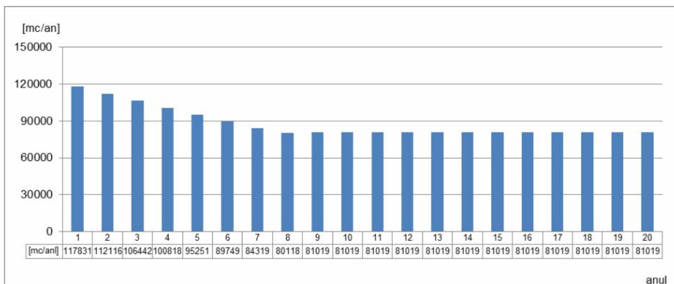
Fig. 3.f – Evoluția consumului de apă în RTS
