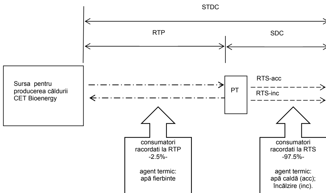
Fig. 1.i - Structura SACC al Municipiului Suceava
