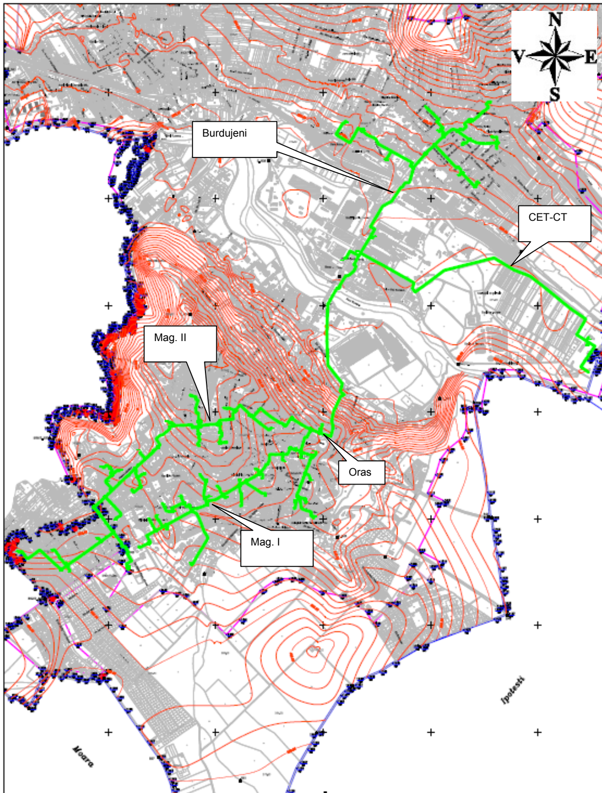
Fig. 1.f – Configurația rețelelor termice primare ale SACC din municipiul Suceava Lungimea de traseu~26.5 km Amplasare: 28% suprateran; 72 % subteran
