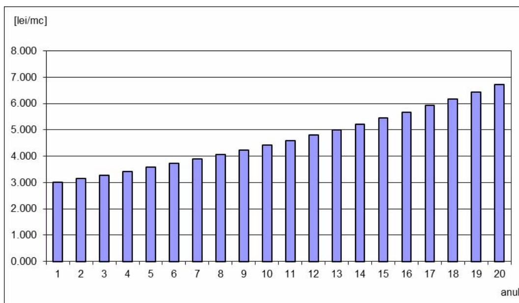
Fig 3.i – Evoluția prețului energiei electrice pentru pomparea în RTS
