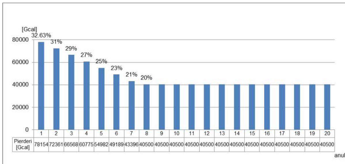
Fig. 3.c – Evoluția pierderilor în sistemul de transport și distribuție
