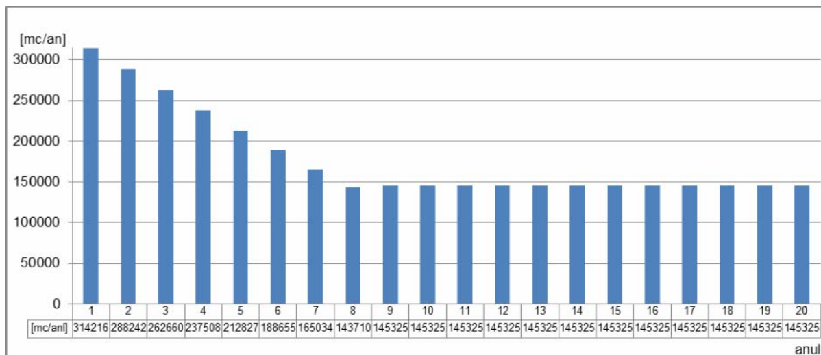
Fig 3.d – Evoluția consumului anual de apă de adaos în RTP
