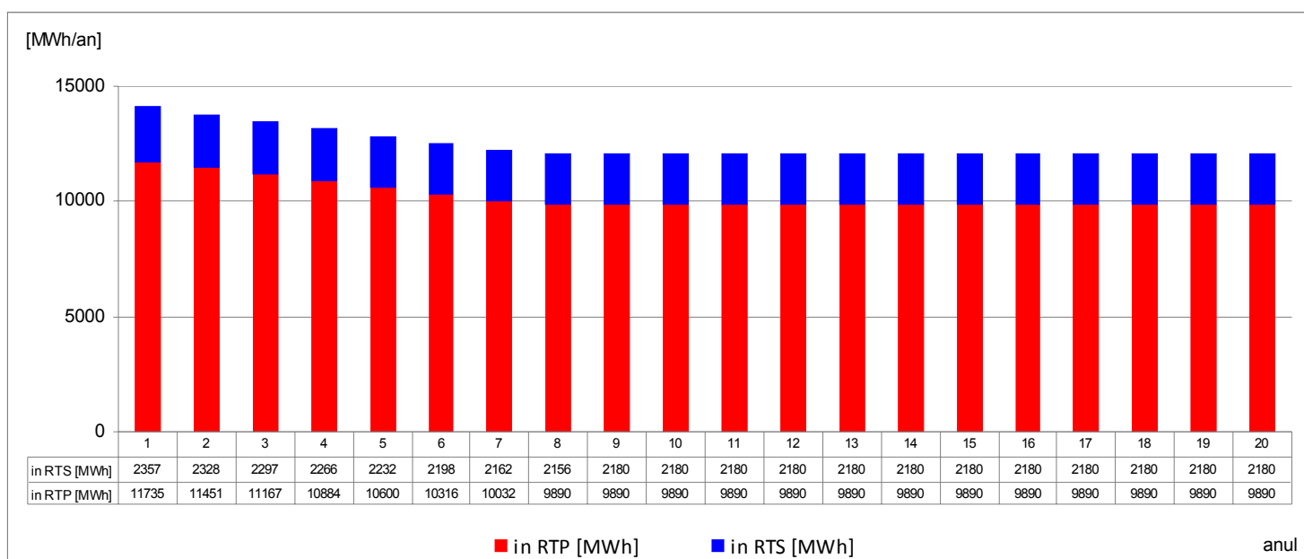
Fig. 3.e – Evoluția consumului anual de energie de pompare
