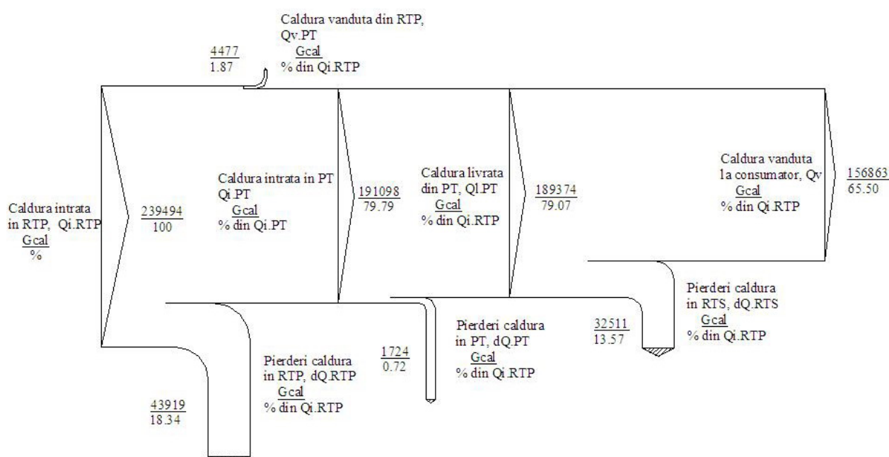
Fig. 1.g – Diagrama Sankey pentru STDC, la nivelul anului 2012
