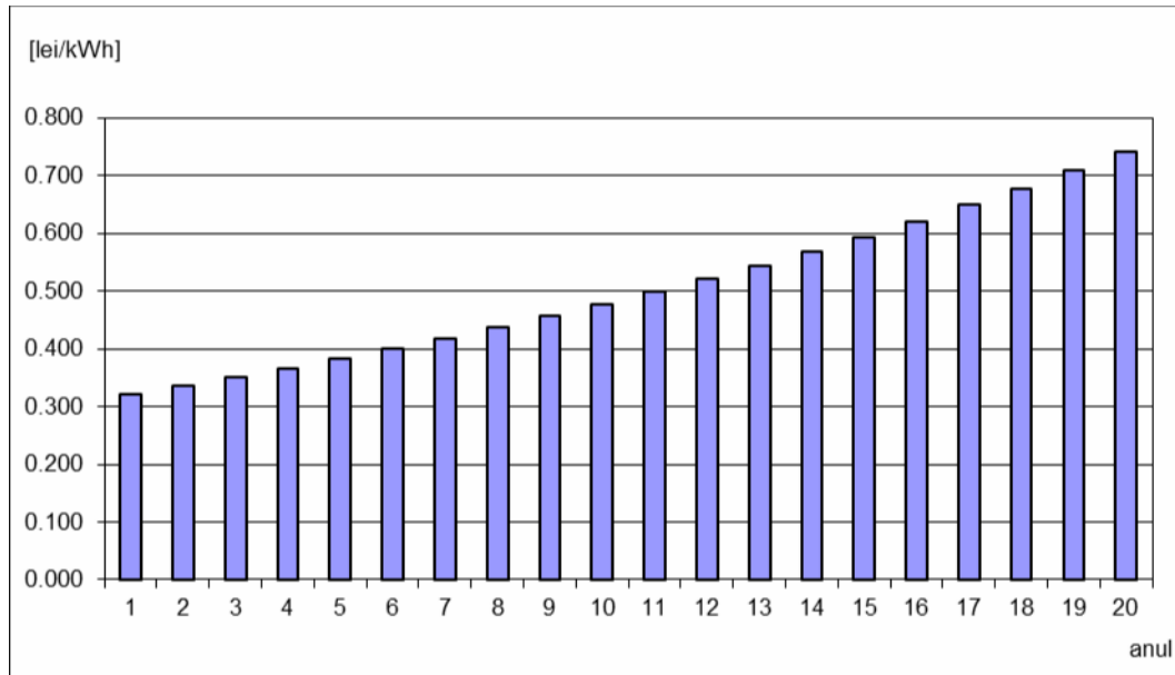
Fig 3.g – Evoluția prețului energiei electrice pentru pomparea în RTP
