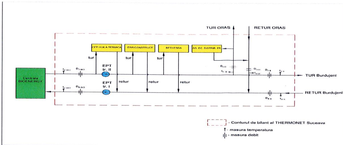
Figura nr. 6: Schema cu punctele și aparatele de măsură a energiei termice la centrala Bioenergy și pe magistralele de apă fierbinte
