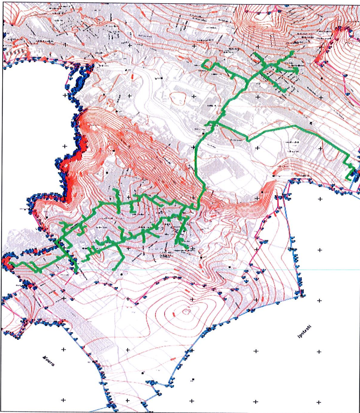
Configurația rețelilor termice primare ale SACC din Municipiul Suceava
