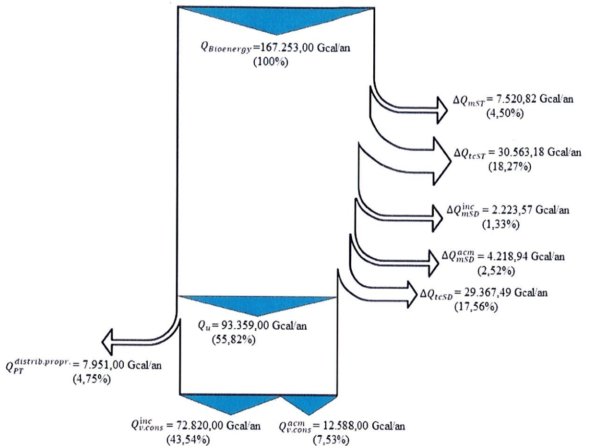
Diagrama Sankey pentru bilantul termoenergetic anual real pentru sistemul de transport și distribuție din municipiul Suceava
