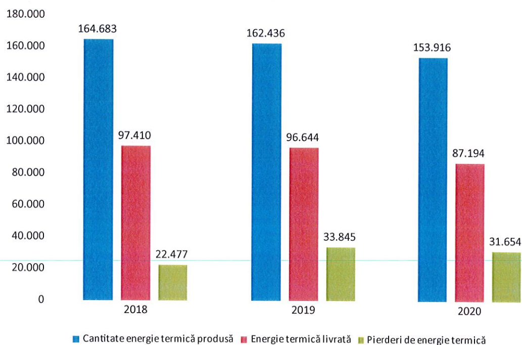
Figura nr. 4: Evoluția cantității de energie termică în rețelele termice secundare și puncte termice [Gcal/an]
