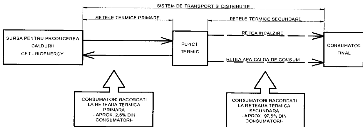
Figura nr. 2: Structura SACET a Municipiului Suceava
