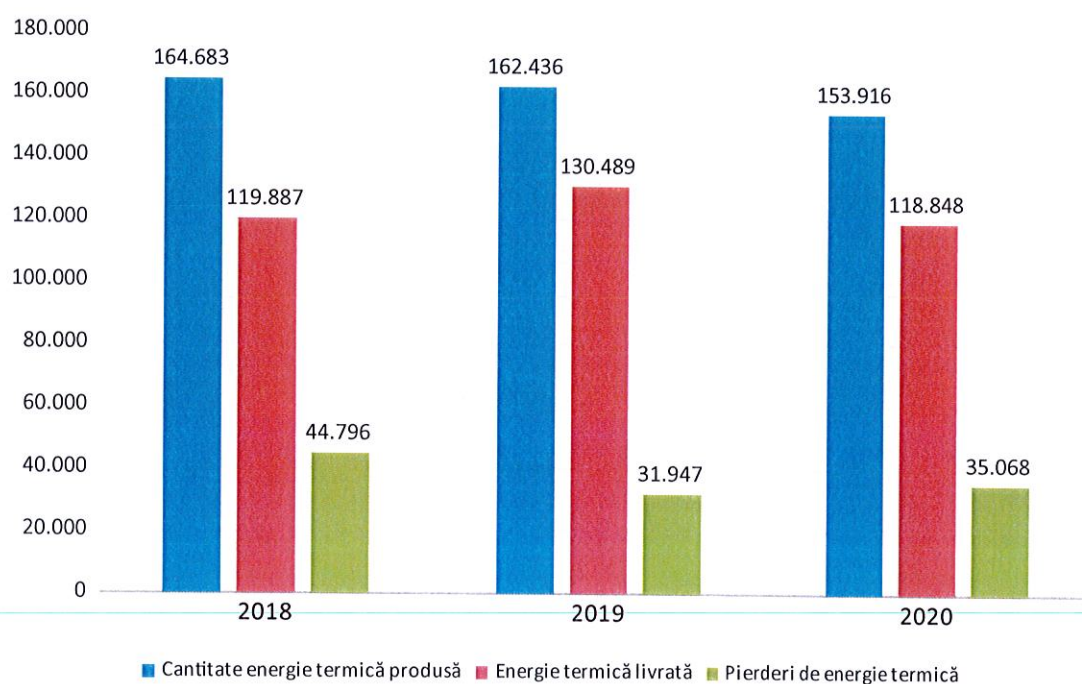
Figura nr. 3: Evoluția cantității de energie termică în rețelele termice primare [Gcal/an]
