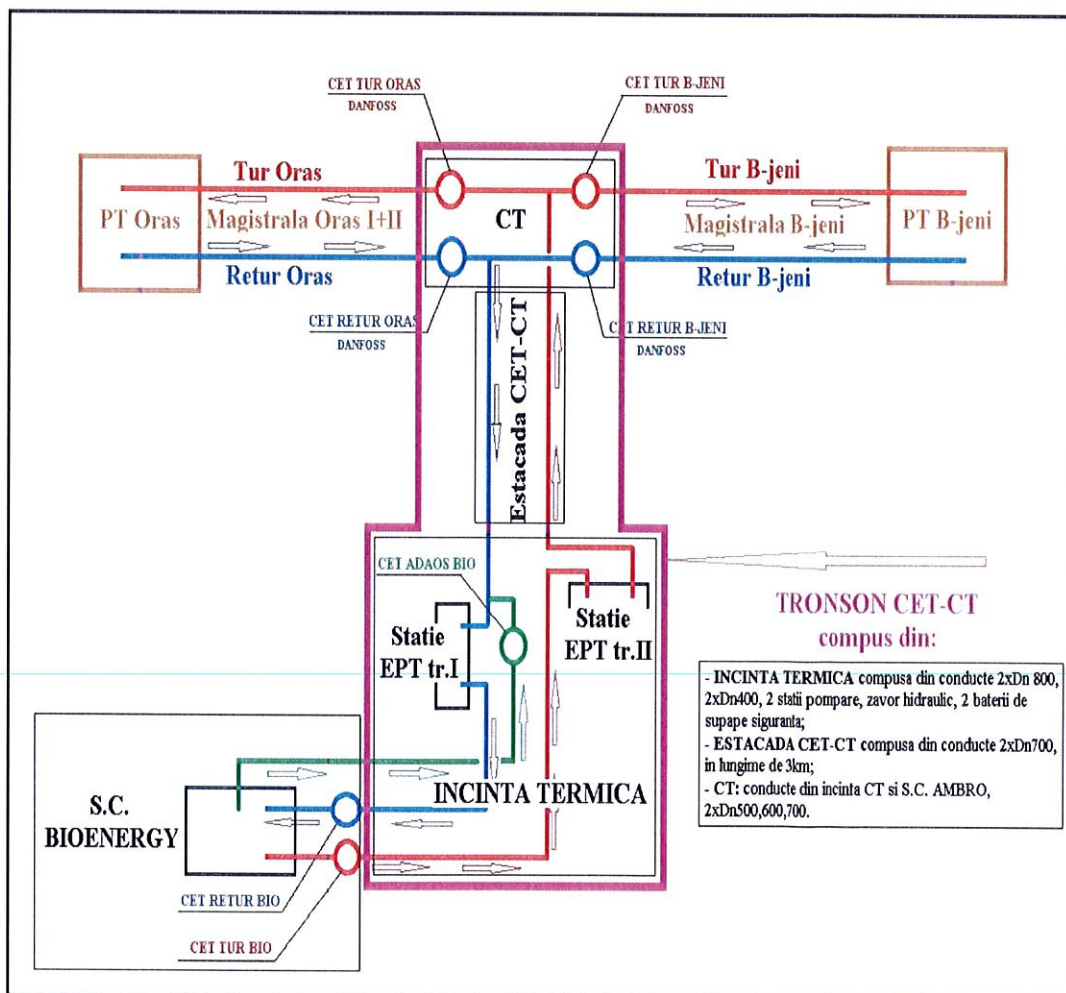
Schema de amplasare a aparatelor de măsurare a energiei termice la producătorul Bioenergy SUCEAVA și pe magistralele de transport apă fierbinte în Municipiul Suceava
