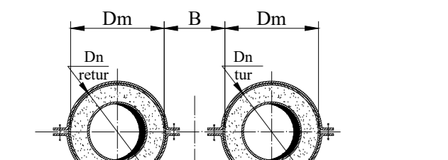
Sectiune transversala conduite termice primare amplasate suprateran - pe stalpi existenti sau nou construiti
