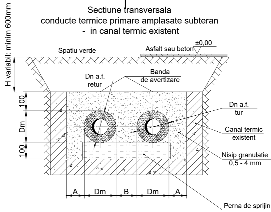
Dimensiuni minime sectiuni transversale conducte primare amplasate in subteran
