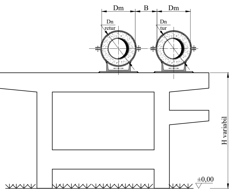
Sectiune transversala conducte termice primare amplasate supraterran - pe stalpi existenti sau nou construiti
