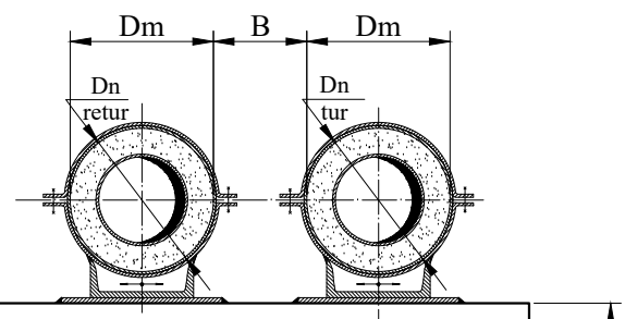
Secțiune transversala conducte termice primare amplasate supraterran - pe stalpi existenti sau nou construiti
