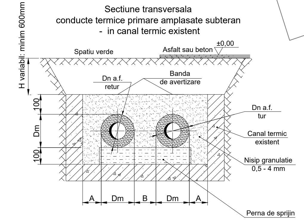
Dimensiuni minime secțiuni transversale conducte primare amplasate in subteran
