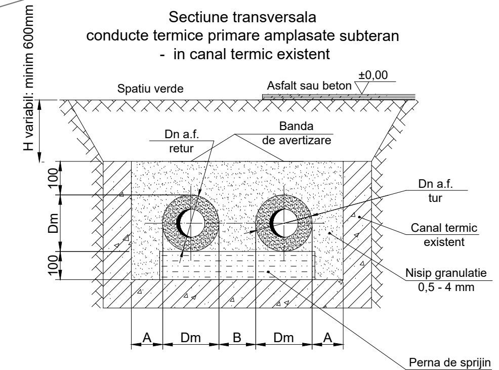
Dimensiuni minime sețiunii transversale conducte primare amplasate in subteran
