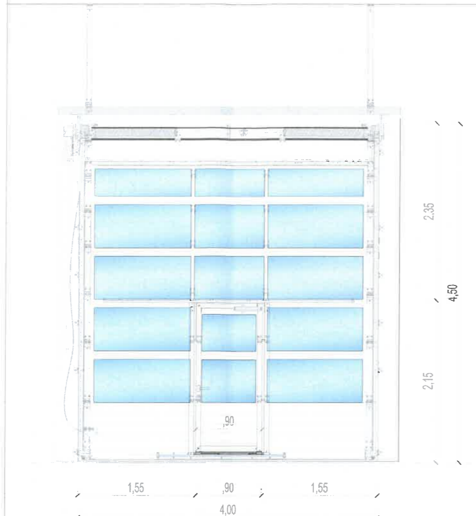
FAȚADĂ INTERIOARĂ UȘĂ SECȚIONALĂ sc. 1_5
