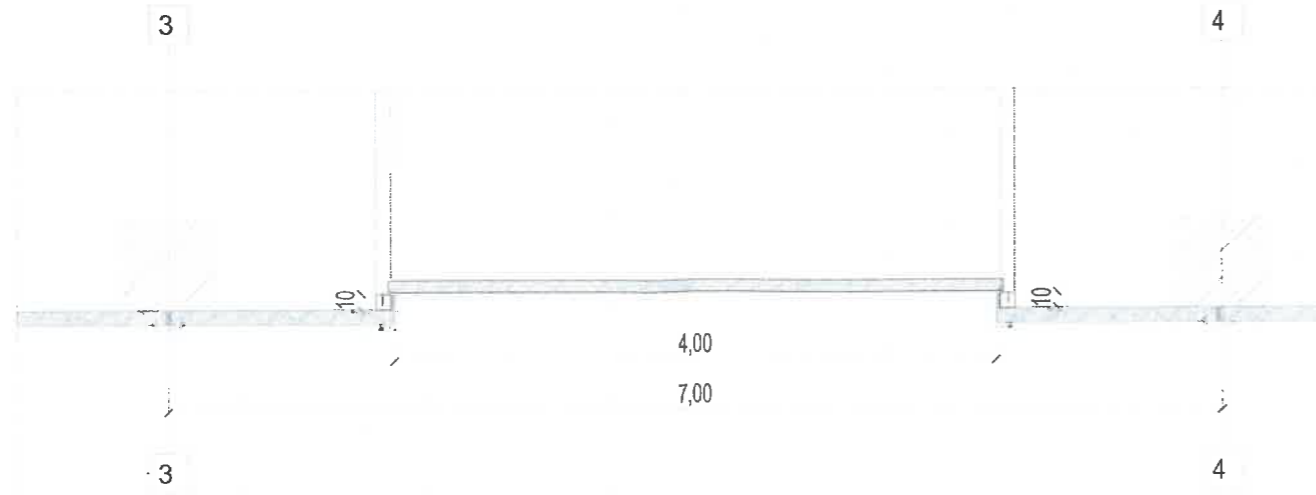
PLAN UȘĂ SECȚIONALĂ sc. 1_50
