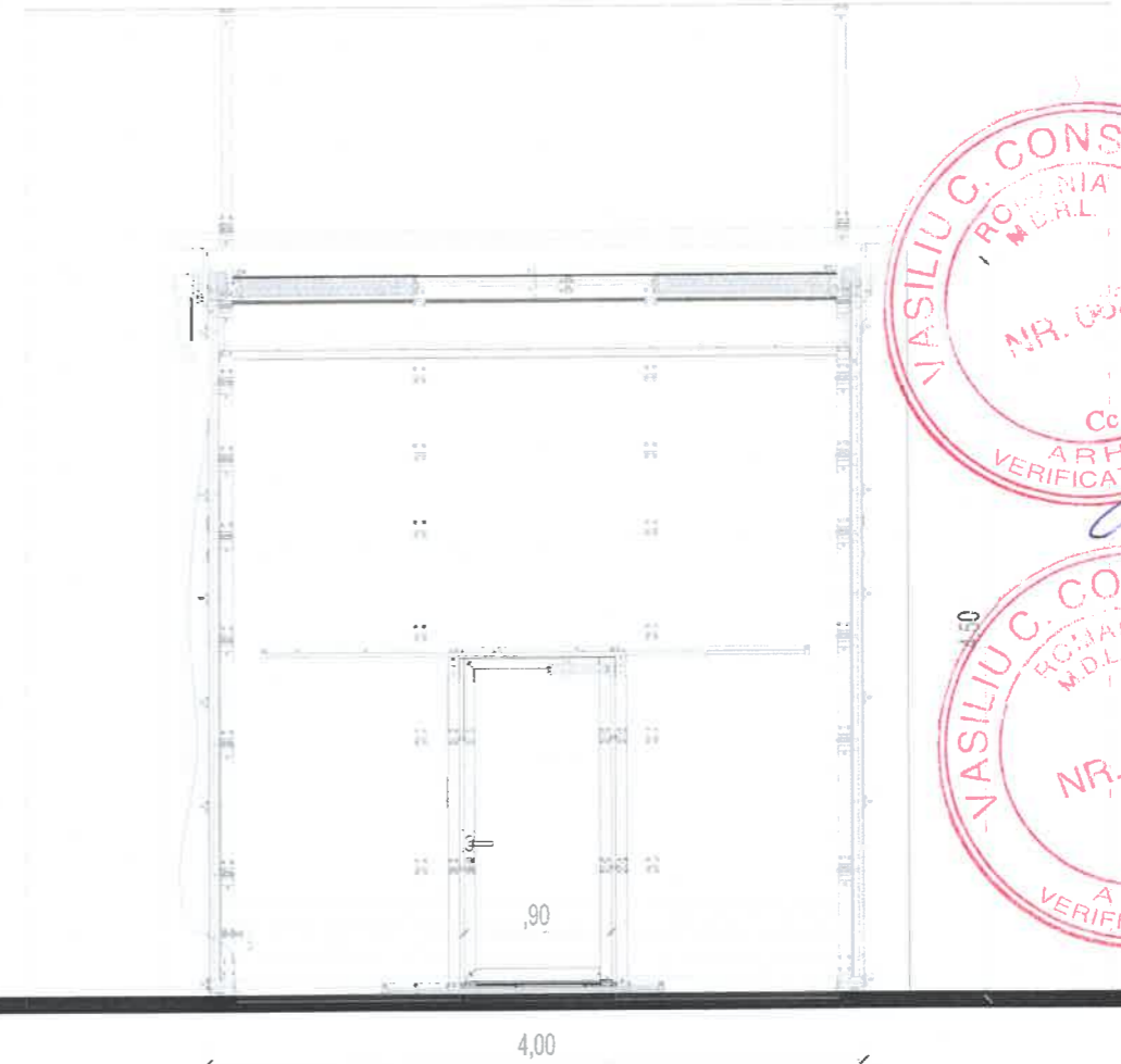
FAȚADĂ INTERIOARĂ UȘĂ SECȚIONALĂ sc. 1_50
