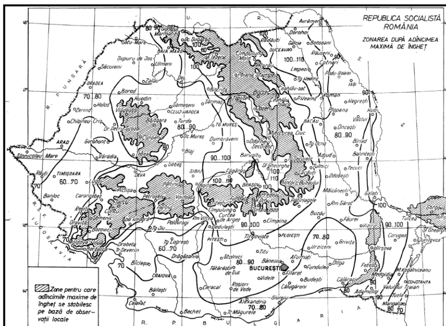
Fig.3.Zonarea după adâncimea de îngheț
