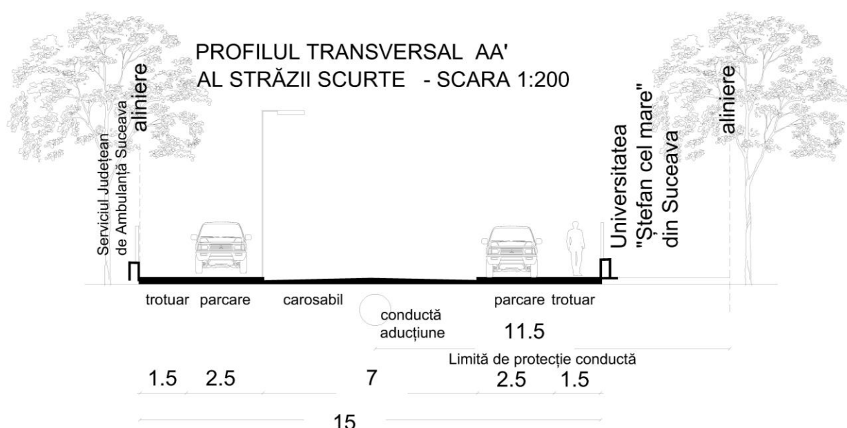
Figura nr. 1 - Extras din documentația de urbanism P.U.G. Municipiul Suceava aprobat prin H.G. nr. 518 din 26 mai 2023
