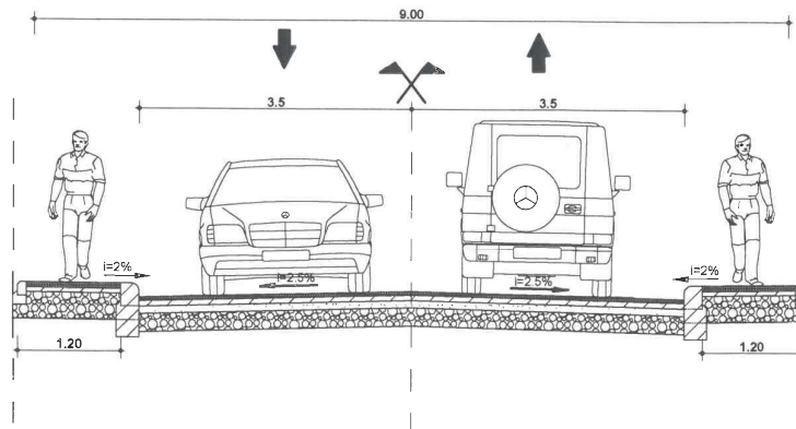
Sectiune 1-1
