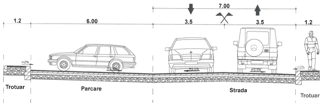
Sectiune 2-2
