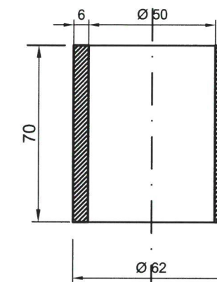
PIESA GURA DE SCURGERE INFERIOARA
