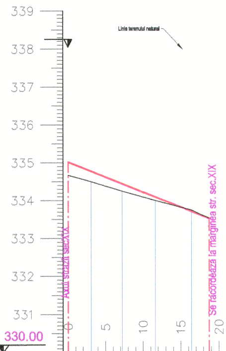
PROFIL LONGITUDINAL Alee granit 1"
