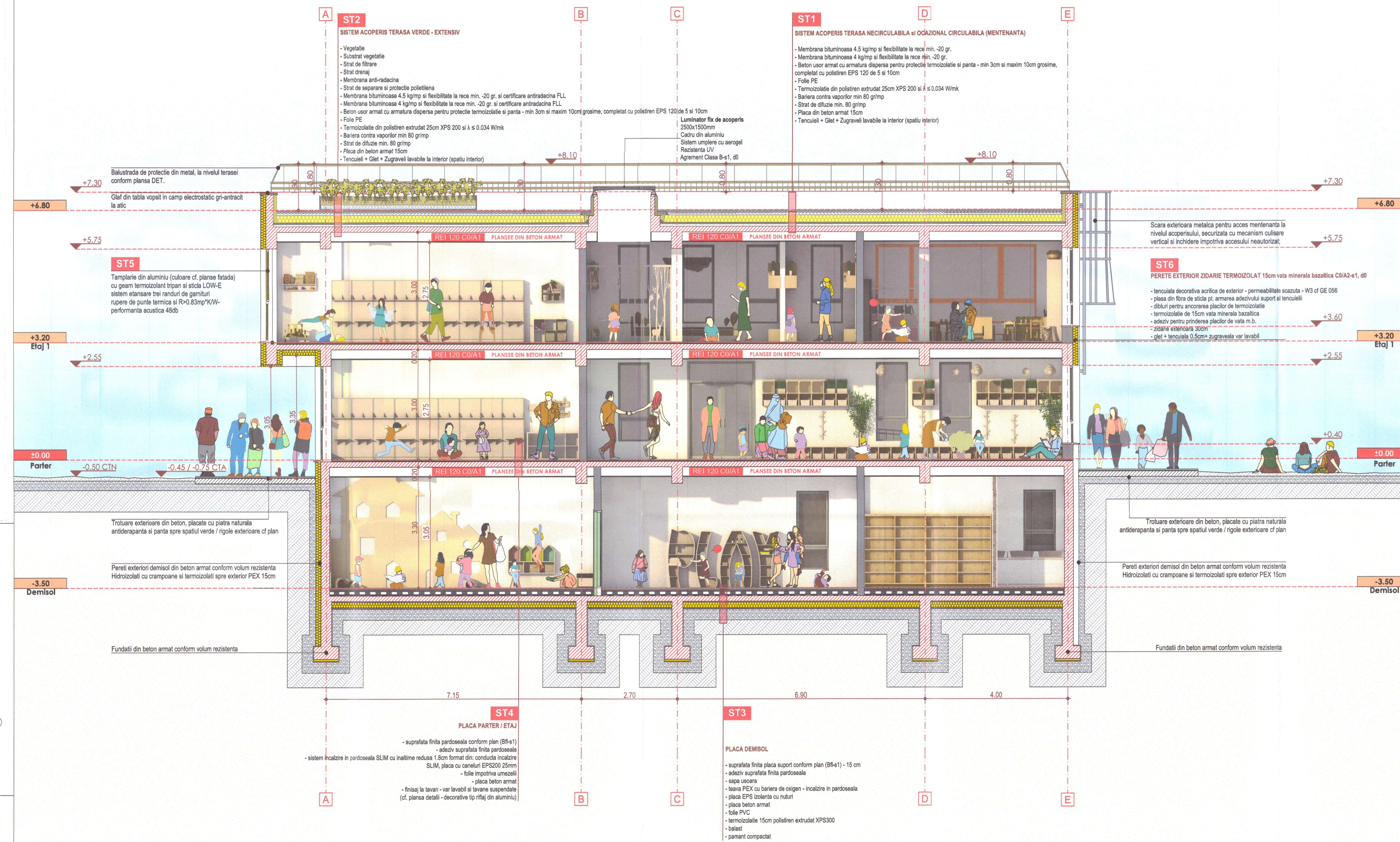
DETALIERE STRATIFICATII PRINCIPALE
