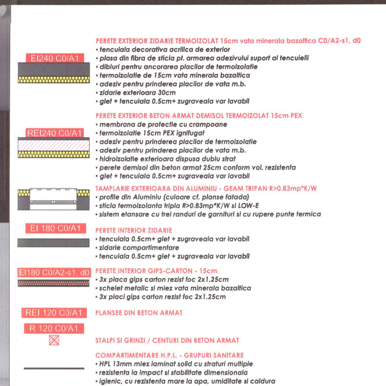
LEGENDA INCHEIDERI SI COMPARTIMENTARI
