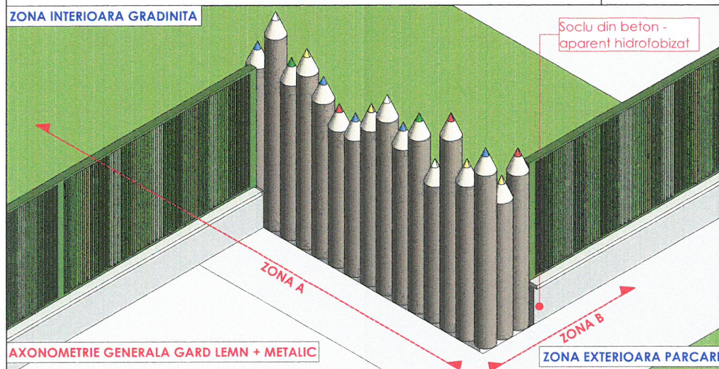
ZONA EXTERIOARA PARCARE
