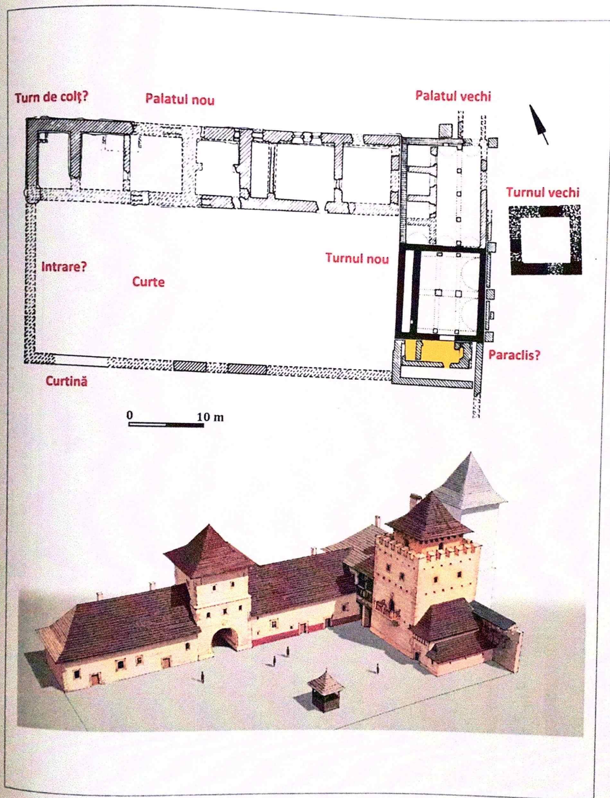
Fig. 20. Planul și reconstituirea curții domnești de la Suceava (autori Adrian Andrei Rusu și Radu Oltean)
