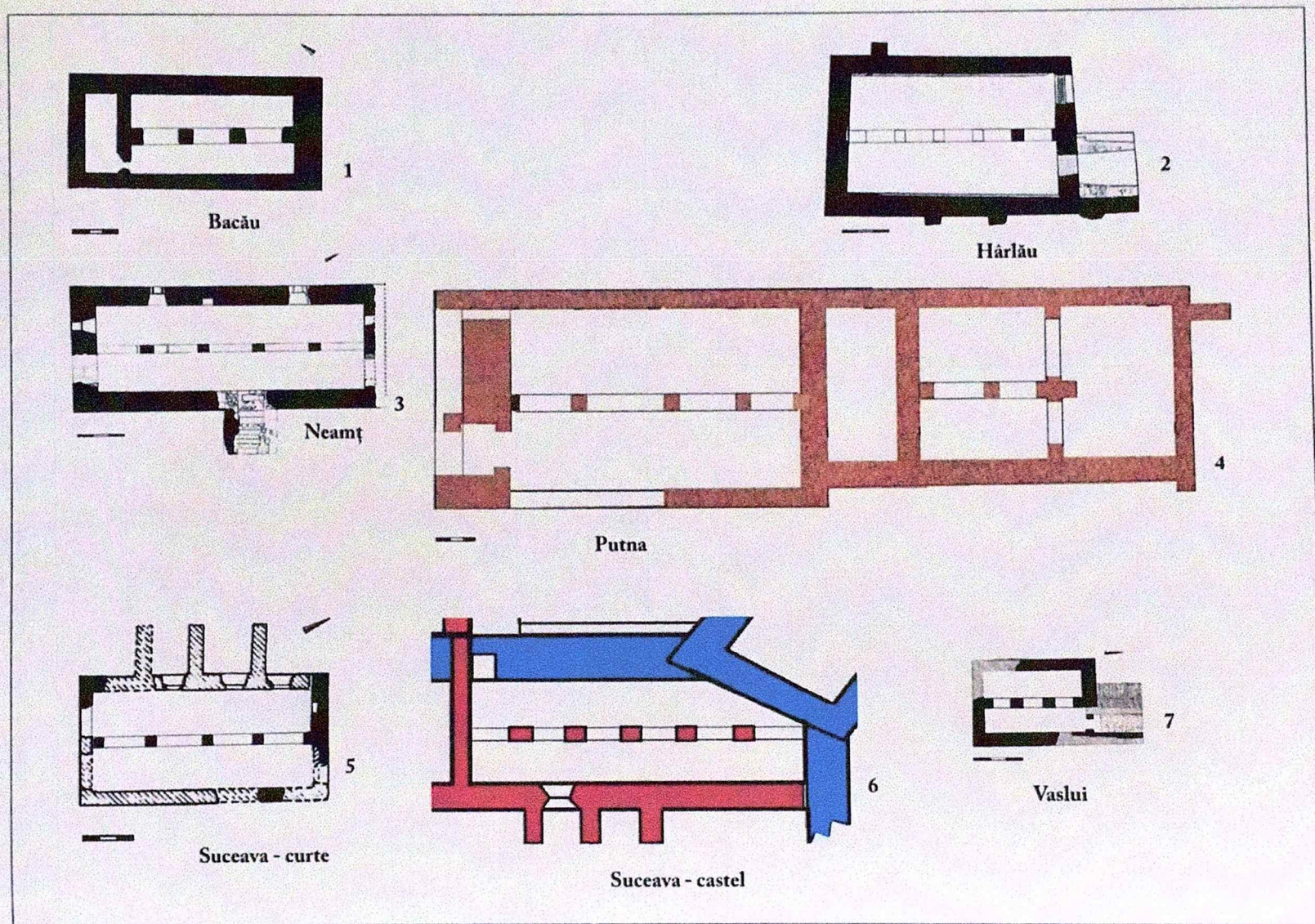
Fig. 21. Pivnițe de palate de la cetăți, curți și mănăstiri domnești: Bacău, Hârlău, Piatra Neamț, Putna, Suceava - curte, Suceava - castel, Vaslui
