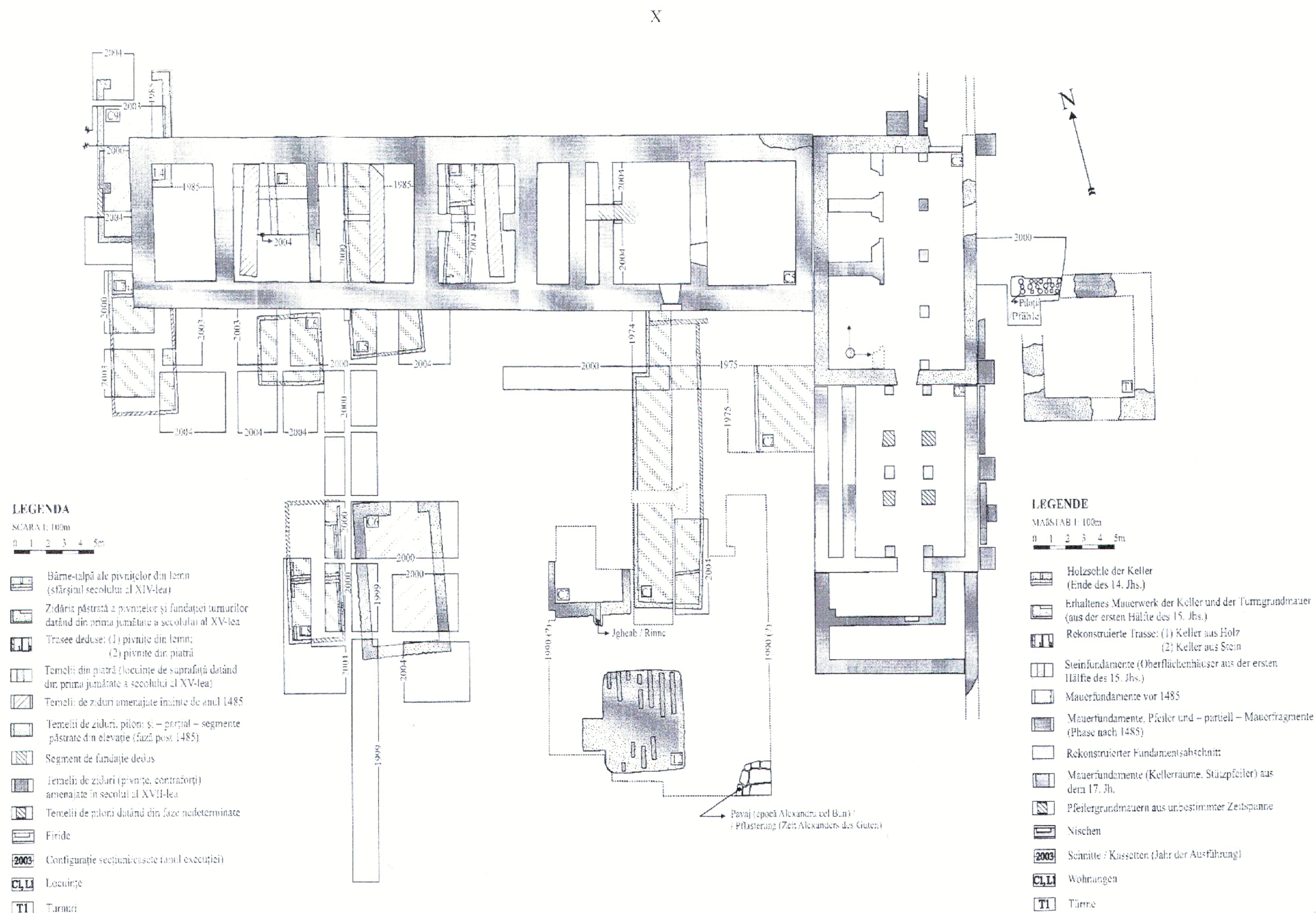
Fig. 9. / Abb. 9. Planul Curții domnești / Grundriss des Fürstenhofs (desen / Zeichnung arh. Gh. Sion)
