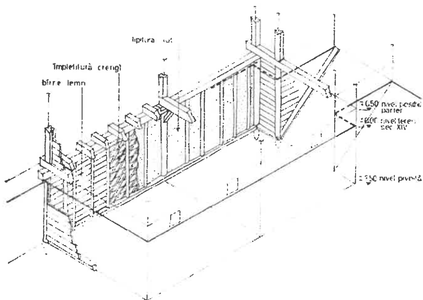
Fig. 11. Propunere de reconstituire a sistemului constructiv al construcției C 1 (perioada domniei lui Petru I) realizată de arh. Gh. Sion (după M. D. Matei, 1989, fig 11)
