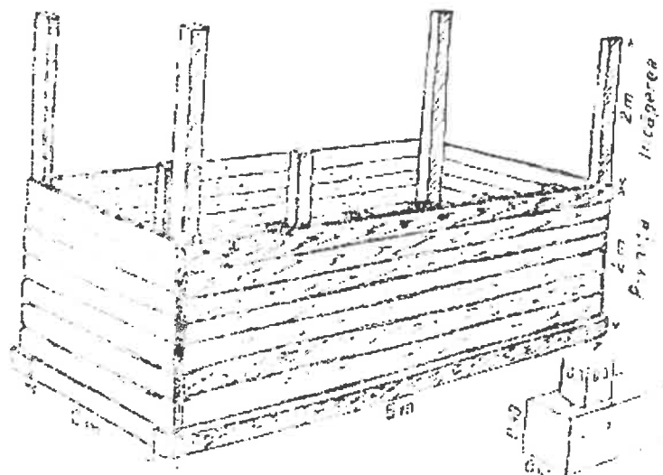
Fig. 9. Descoperirea pivniței nr. 1 și reconstituirea ei (Gh. Diaconu, SMIM , I, 1956, fig. 2, 4).
