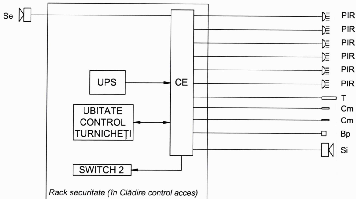
Clădire control acces - Cameră tehnică
